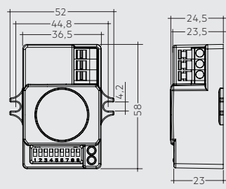
smartSWITCH HF 12DP MB S f (28003499)
