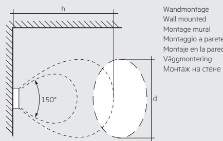
smartSWITCH HF 12DP MB S f (28003499)
