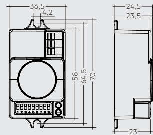
smartSWITCH HF 12DP MB f (28003498)
