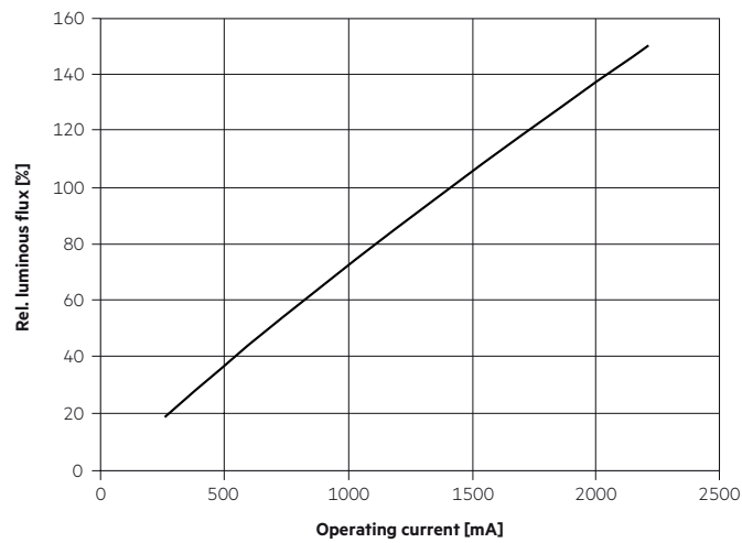
SLE G7 21mm 6000lm xxx EXC
