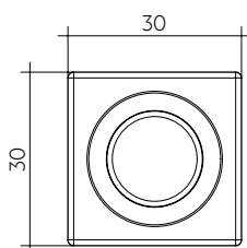
MSensor G3 SFI 30 PIR 10DPI WH
